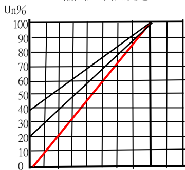
Low limit setting 輸出量下限設定
